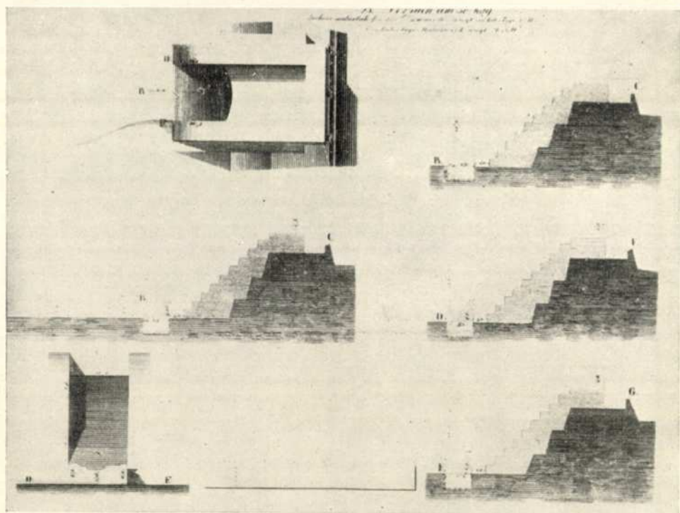
Földnyomás-kísérlet. Mártony: „Versuche über den Seitendruck der Erde” c. könyvéből (1828)
