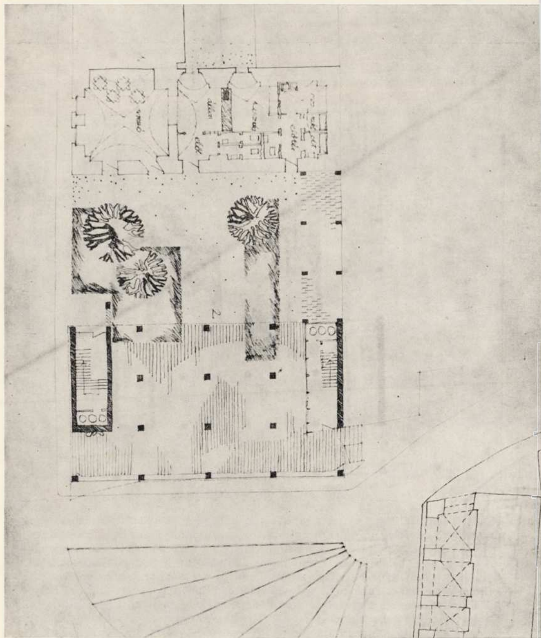
4. Az Orsolya tér 4. sz. épület újraépítése — földszinti alaprajz (Balról a csatolt Fegyvertár u. 2. sz. épület)
