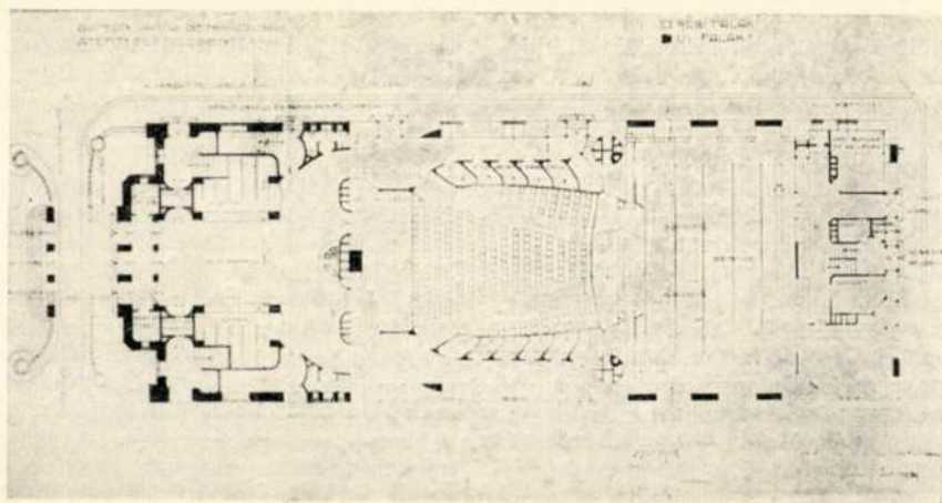
A színház tervének földszinti alaprajza
