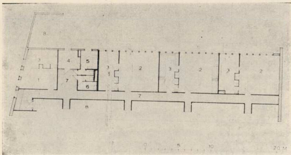
A II. emeleti (tetőtéri) alaprajz: 1. két férőhelyes műterem, 2. négy férőhelyes műterem, 3. két férőhelyes háló, 4. főzőfülke, 5. női fürdő, 6. férfi fürdő, 7. közlekedő, 8. tetőtér
