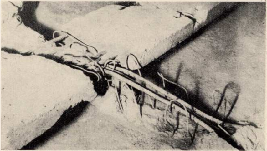
A vasbeton erkélyszerkezet szabaddá vált vasbetétei
