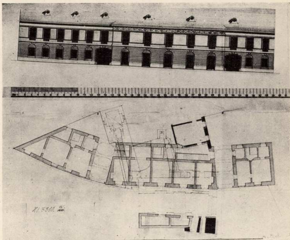
2 A Hátsó kapu lebontásának II. sz. terve. Az előző képen látható ház nagyobbított megoldása. A belső városfalra vivő lépcső és az órség szobája is megsemmisült
