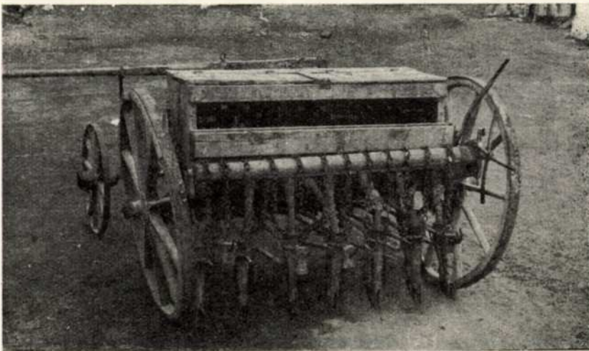
A Bokor-féle vetőgép. Lex József tulajdona Nagycenken
