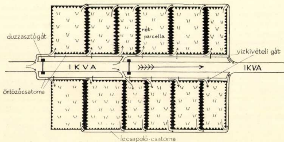
Az öntözési rendszer vázlatja. Lovas Gyula rajza
