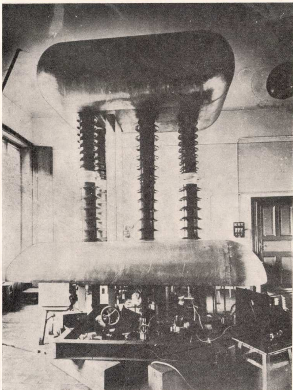
Van de Graaff-generátor a Soproni Műszaki Egyetemi Karok Elektrotechnikai tanszékén 1951-ben. Diebold Károly felvétele
