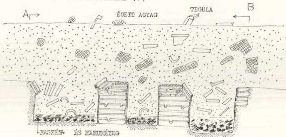
6. A fertőrákosi tégláégető kemence
