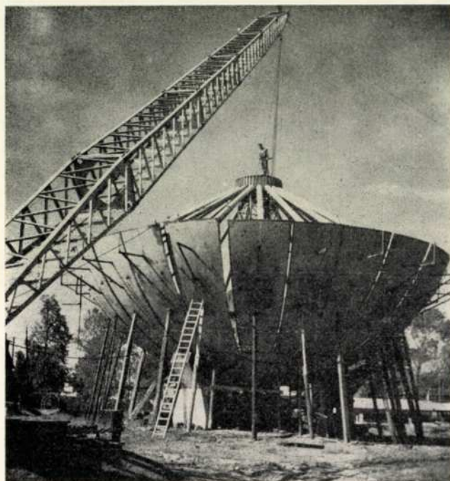
18. A gömbgáztartó szerelése (1965)
