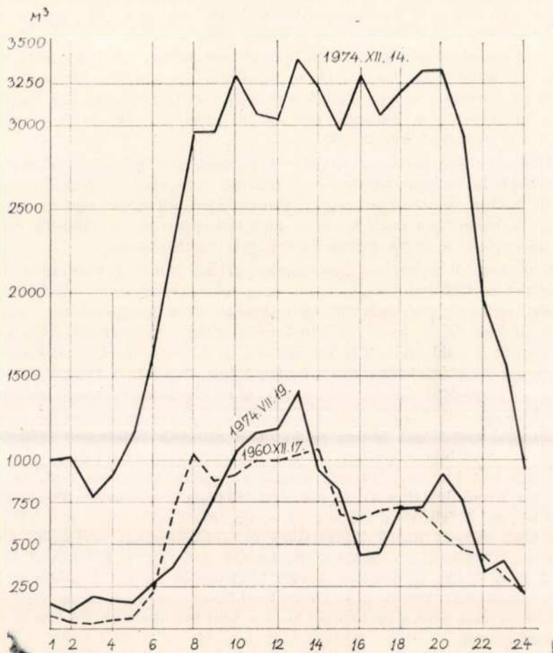
34. Óránkénti gázleadás egy-egy decemberi (1960, 1974) és egy júliusi hétköznapon (1974)
