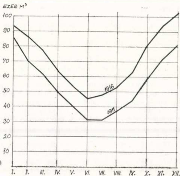
8. Havonkénti gázleadás 1911-ben és 1916-ban
