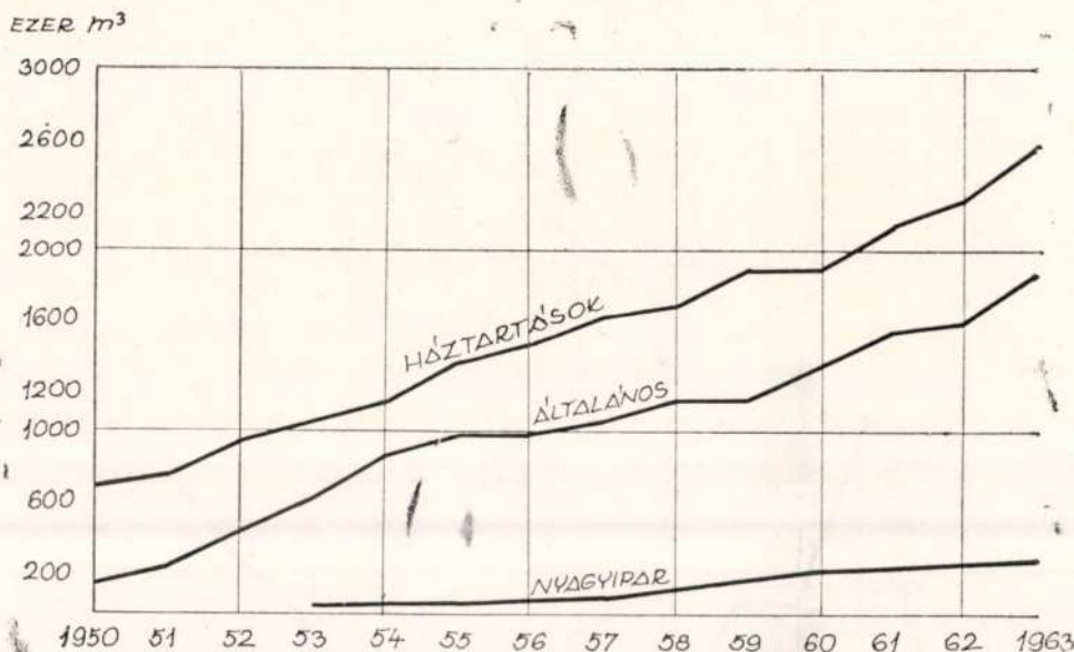
30. A gázfogyasztás megoszlása (1950—1963)
