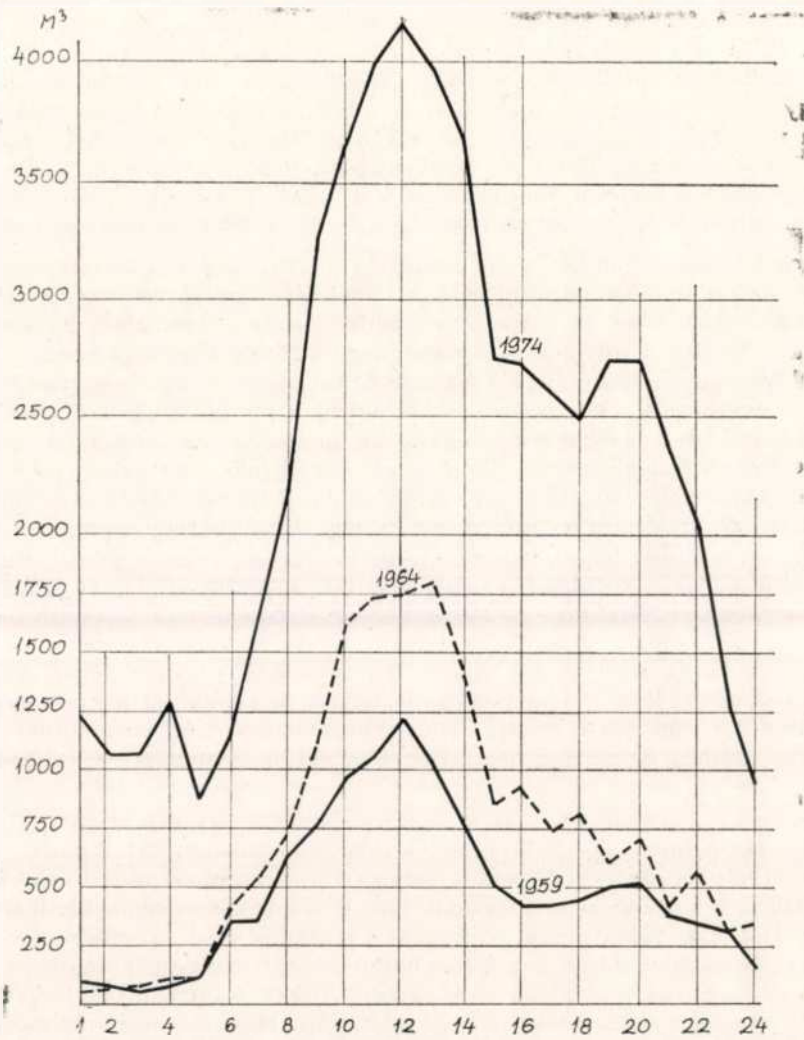
33. Óránkénti gázleadás egy-egy decemberi vasárnapon (1959, 1964, 1974)
