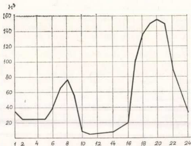
5. Óránkénti gázleadás 1874. jan. 16-án
