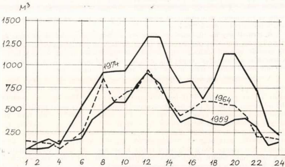
32 b. Óránkénti gázleadás egy-egy júliusi hétköznapon (1959, 1964, 1974)
