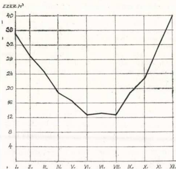
6. Havonkénti gázleadás 1874-ben
