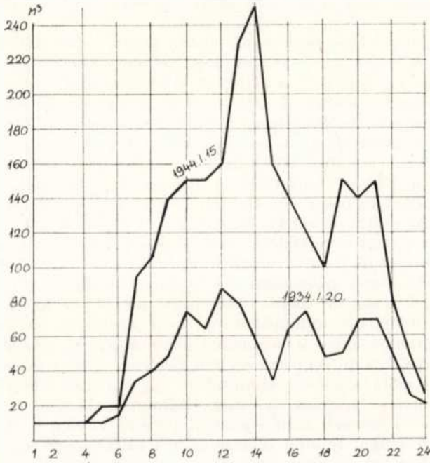
32 a. Óránkénti gázleadás (1934, 1944)
