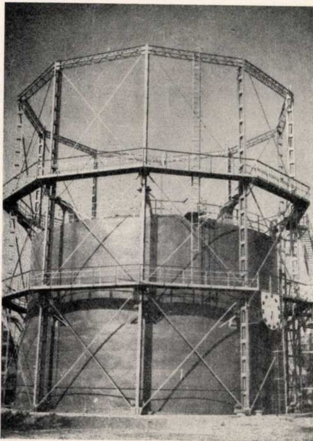
16. Az új, 4500 m 3 -es gáztartó (1955)
