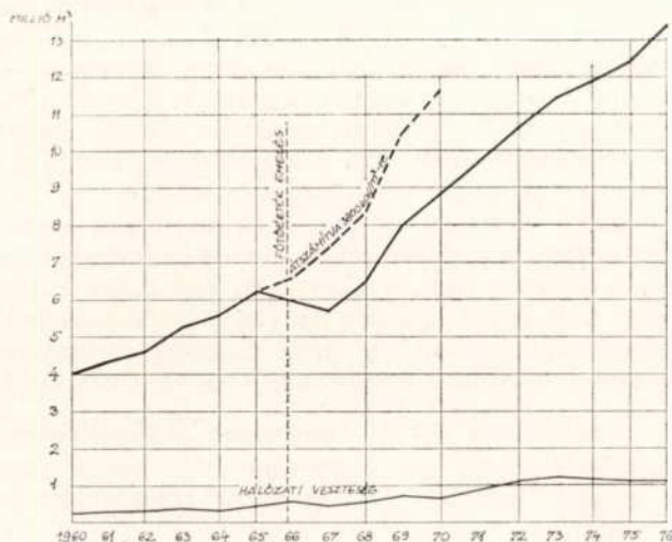
21. A gáztermelés az 1960—1976. években
