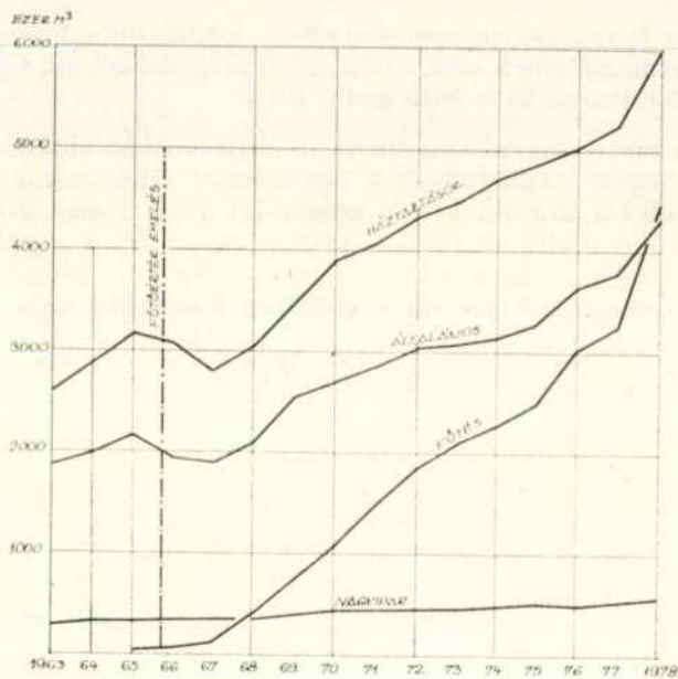
31/a. A gázfogyasztás megoszlása (1963—1978)
