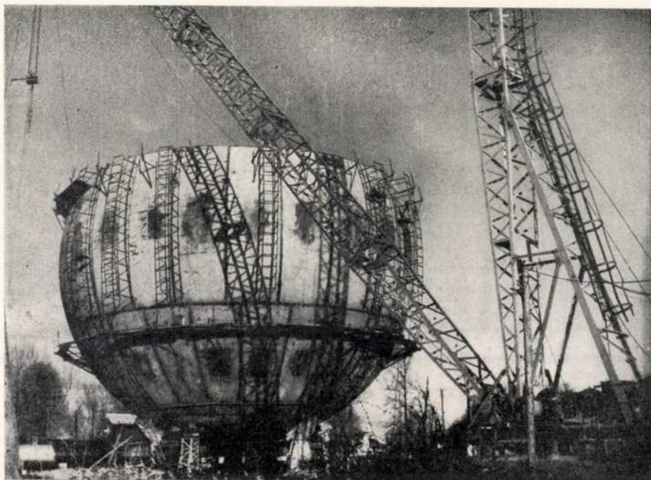
19. A gömbgáztartó szerelése (1965)
