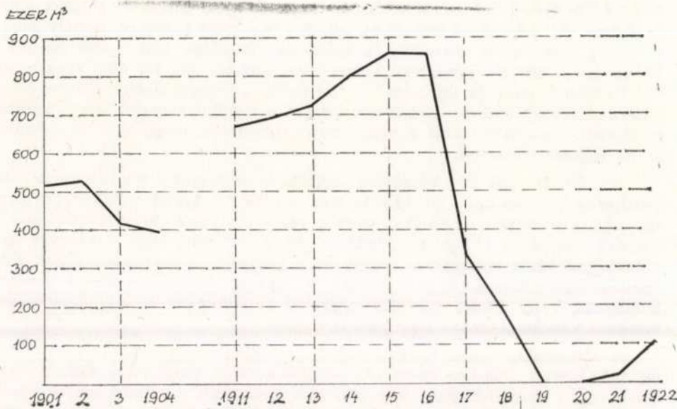
7. Gáztermelés az 1901—1922. években
