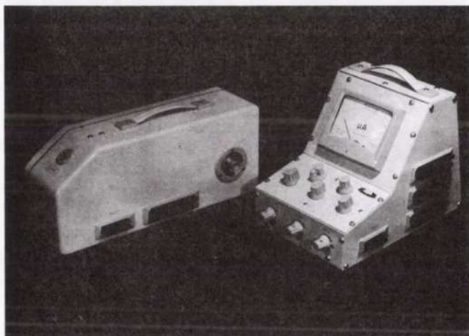
17. Az MTV-2 mágneses érzékelő és tápegysége.
