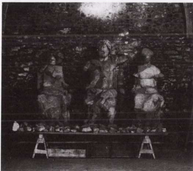
A kapitoliumi triász felállítása a Fabricius-ház római kőkiállításába. Szakál Ernő rekonstrukciója, munkaközi felvétel.
