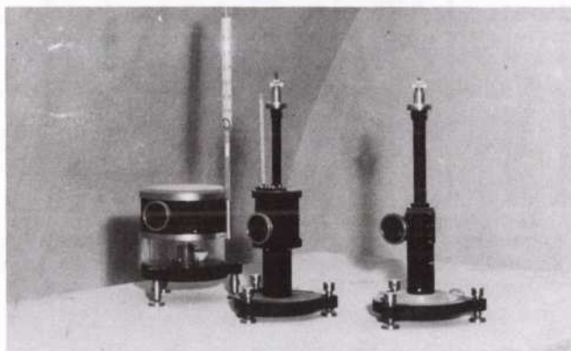
8. Az obszervatórium La Cour-rendszerű mágneses műszerei, amelyek 1961-től napjainkig működtek.
