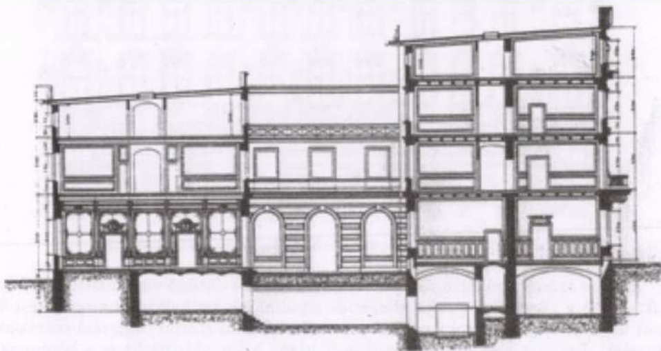
9. A felépült ház metszete a tetőfedés megoldásával.
