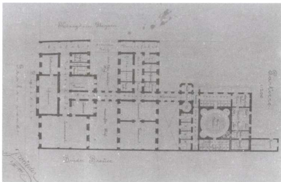
4. Wälder József rajza a szálloda "fürdős" változatának földszinti alaprajza (1891)
