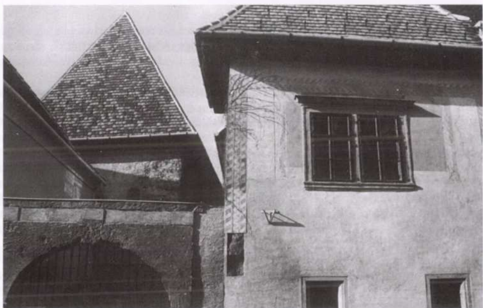
20. Középkori zsinagóga műemléki helyreállítása az Új utcában. 1972. Sedlmayr János (OMF) építész terve.
