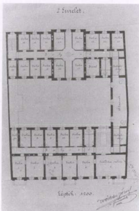
5. Wälder József rajza a szálloda végleges alaprajzáról (1894).
