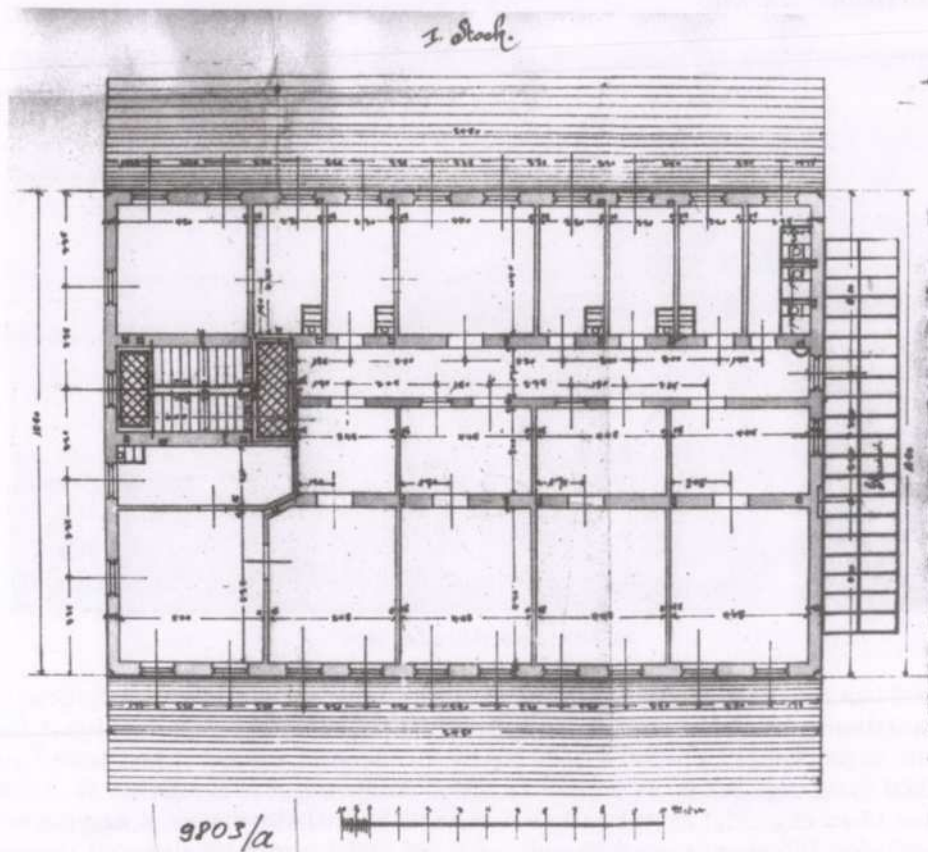
13. Szálloda a Lővészkerthez emeleti alaprajza (Gerhard F. Benesch 1898. elpusztult).
