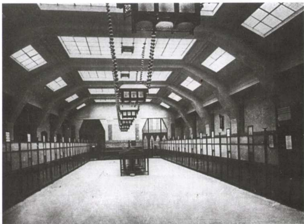
2. Polygonális vasbeton-keretszerkezet mint a belső teret meghatározó architektúra a posta felvételi termében. 1913. Orth Ambrus és Somló Emil építészek terve.
