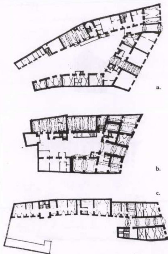
2. Soproni vendégfogadók alaprajzai: a.) Ötvös utca 19. „Arany kakas” fogadó b.) Ötvös utca 9. sz. „Zöld fa” fogadó, c.) Várkerület 51. „Arany Angyal” fogadó
