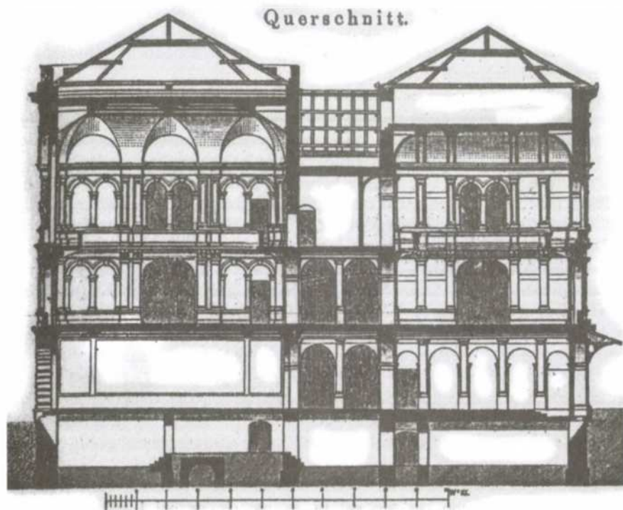
2. kép Tervezett keresztmetszeti kialakítás (Ludwig Wächtler terve)
