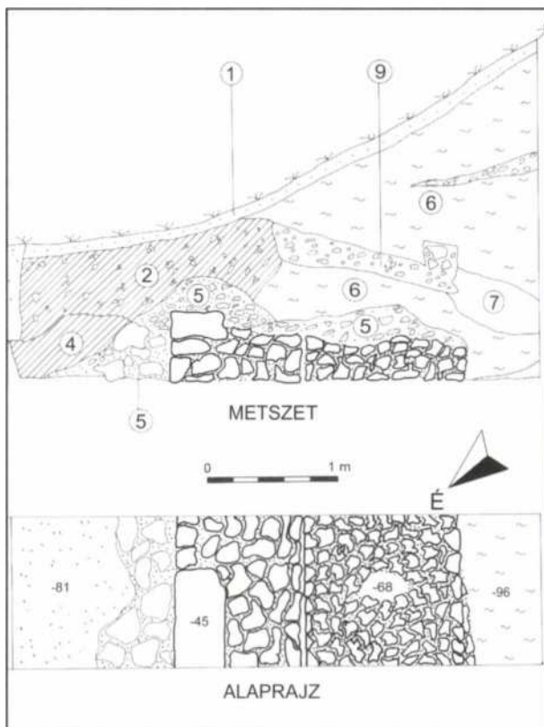
10. kép. A két periódusú pódiumfal alaprajza és metszete a 24. kutatóárokban. 1. humusz, 2. sűrű föld kövekkel, 4. sűrű föld, 5. kőomladék rétegek, 6. agygrétegek, 7. homok, 9. apró kötőrmelések.
