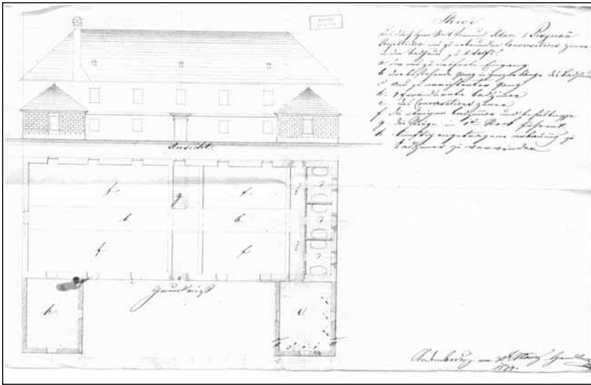
10. ábra. Balfi fürdő alaprajza és homlokzati rajzának részlete 1833. (MNL GyMSM SL, SVLt, XXV. 5220)
