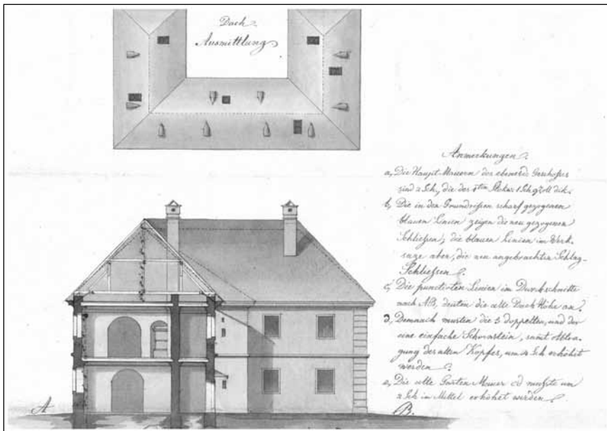
3. ábra. A Soproni Közkórház homlokzati és alaprajza, 19. sz. első fele (MNL GyMSM SL, SVLt, VIII. 918.)
