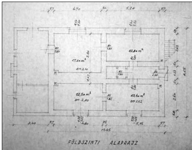
12. kép. Az épület jelenlegi földszinti alaprajza
