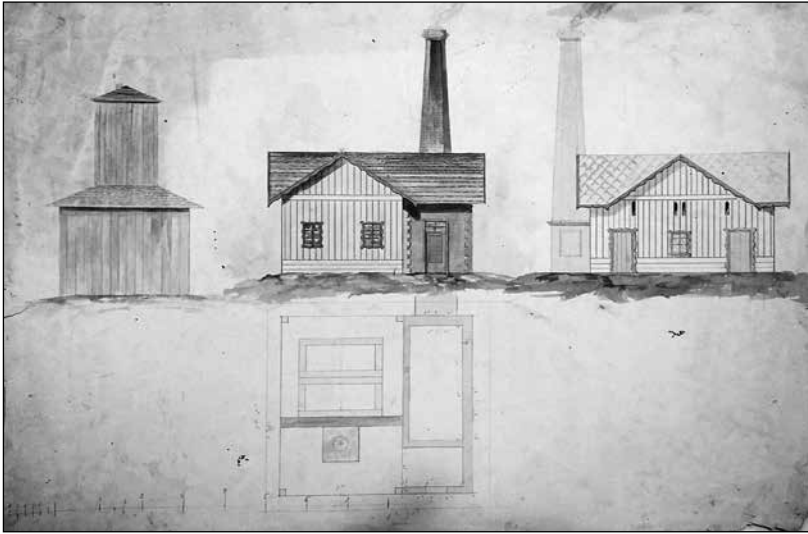
11. kép. A brennbergi gépház akvarellal színezett vetületi- és alaprajza
