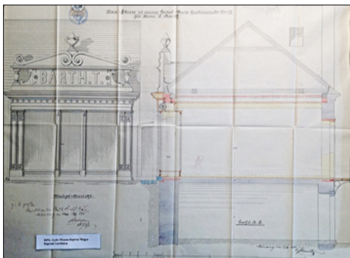
13. kép. A Várkerület 28. számú épület átépítésének második, megvalósult terve (MNL GYMSV SL XXIV. 8239.)
