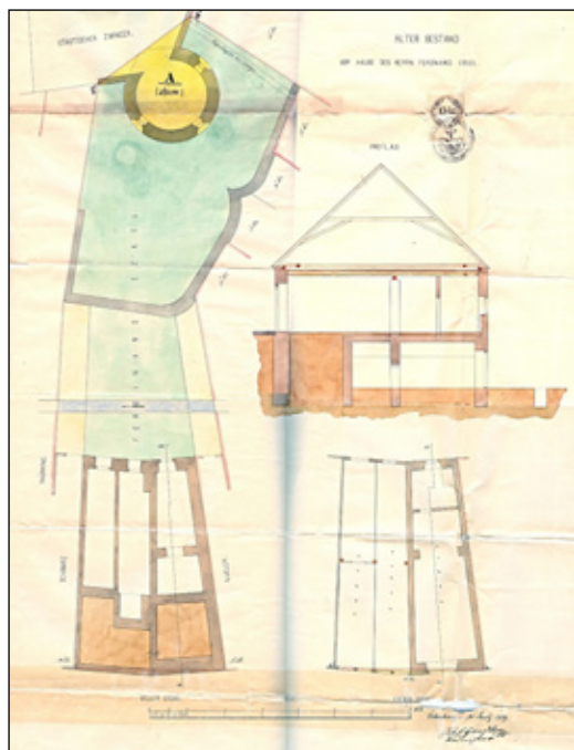
7. kép. Handler felmérési terve a korábbi két, földszintes épületről 1859-ből és a beépítendő telek (MNL GYMSV SL XXIV. 5153.)
