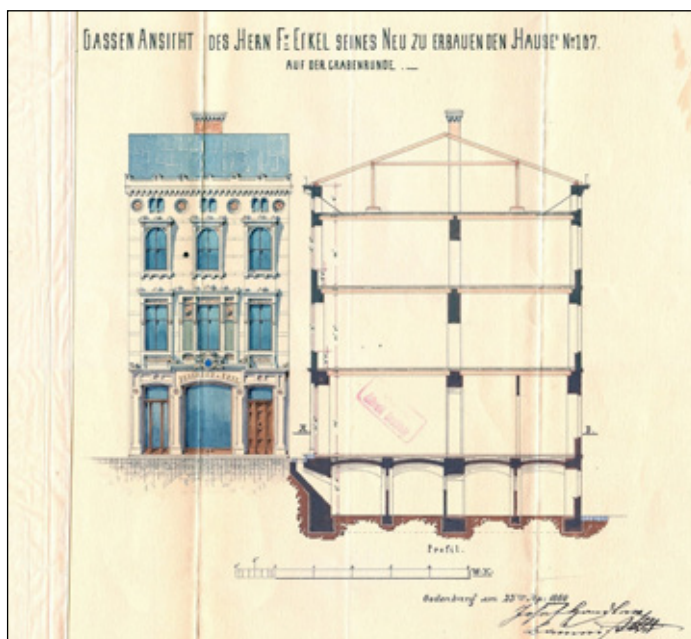
8. kép. A Várkerület 56. számú épület utcai homlokzata és metszete 1860-ból (MNL GYMSV SL XXIV. 5153.)
