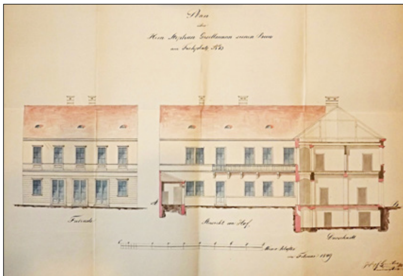
3. kép. A Várkerület 6. számú épület utcai homlokzatának és udvari bővítésének tervlapja 1849-ből (MNL GYMSV SL BC 14/1849.)
