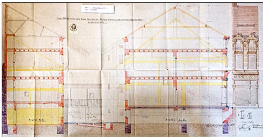
12. kép. A Várkerület 86. számú épület 1876-os átépítésének hosszmetSZete és homlokzati rajza (MNL GYMSV SL XXIV. 8039.)
