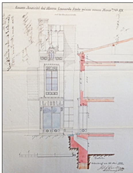
9. kép. A Várkerület 64. sz. új épület tervezett utcai homlokzata és metszetének részlete (MNL GYMSV SL XXIV. 5180.)
