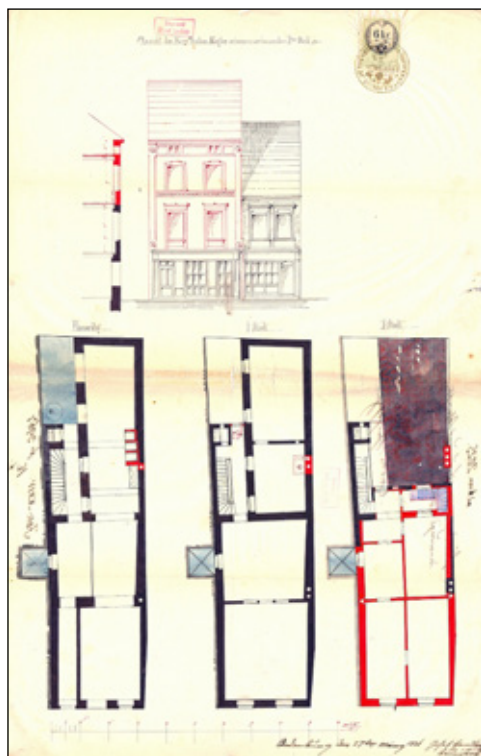
4. kép. A Várkerület 115. számú ház II. emelettel való bővítésének 1856-os tervrajza (MNL GYMSV SL XXIV. 3967.)
