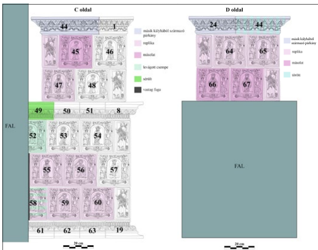
8. kép. A kályha C oldala. Levágott: 52, 58. Sérült: 49. Cserélt: 44. Másolat: 45. Replika: 47, 55-56, 59-60, 65. (Rajz: Rakonczay Rita)
