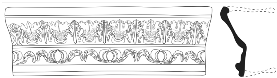
20. kép. Párkánycsempe III. típus. A párkányelem a kályha tetejét lezáró koronázó párkány. (Rajz: Rakoncay Rita)
