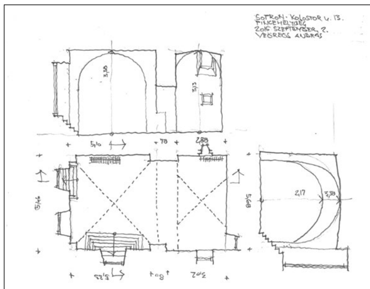
4. kép. A helyiség felmérési rajza
