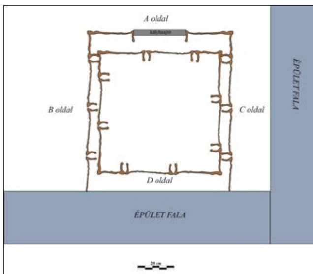
5. kép. A kályha alaprajza. Rajz: Rakonczay Rita
